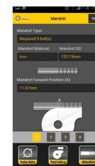
Posición del mandril
