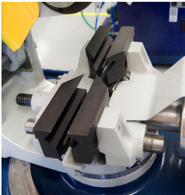
Mordazas automáticas autocentrables.
